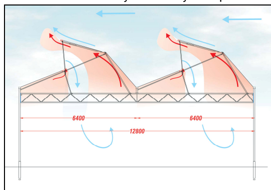
Serre Venlo système asymétrique
