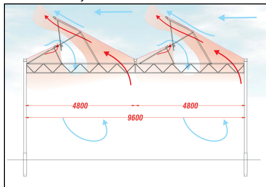
Serre Venlo système demi-ventilation déflecteur
