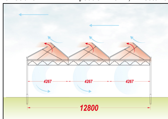
Serre Cabrio Air 2000 poutre 12800, 1 coté ouvert
