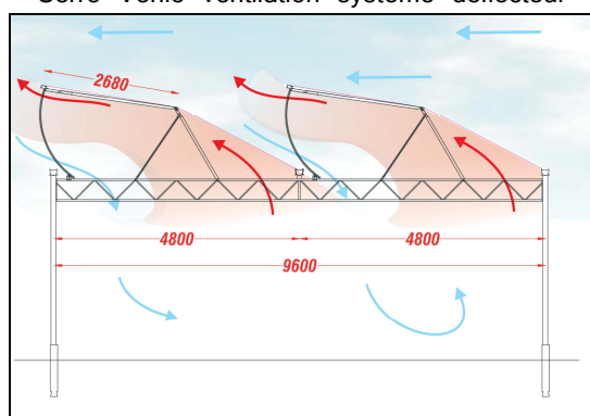
Serre Venlo ventilation système déflecteur
