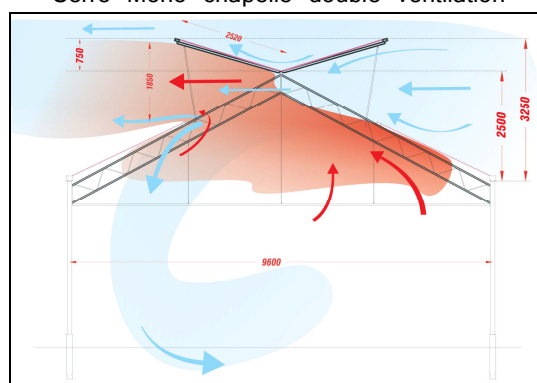
Serre Mono-chapelle double ventilation
