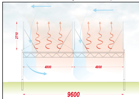
Serre Cabrio 2000 poutre 9600, ouvert
