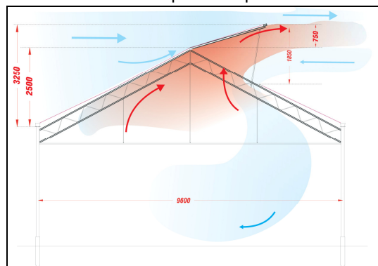
Serre Mono-chapelle simple ventilation
