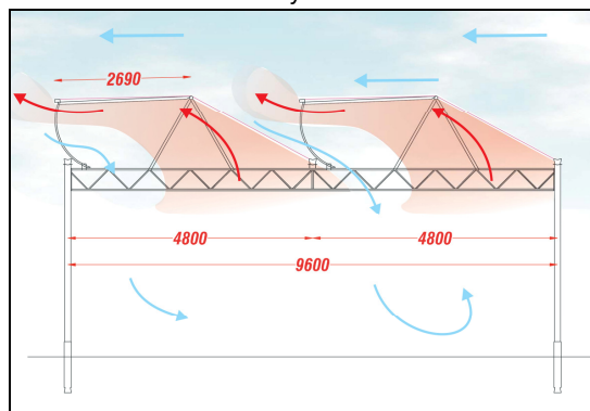
Serre Venlo système standard
